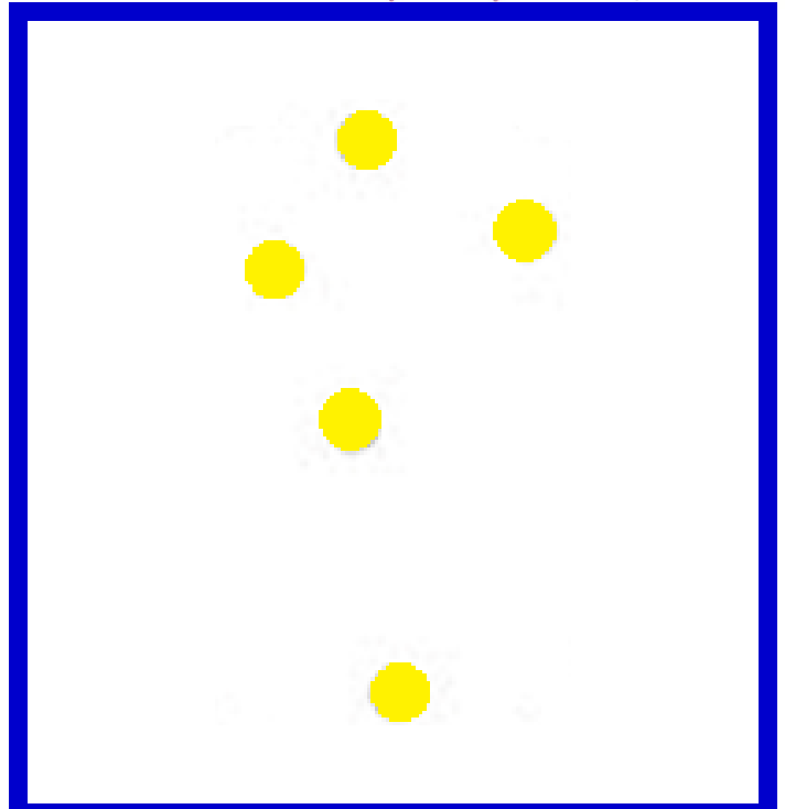
El Boyero
