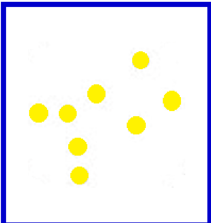
Géminis
