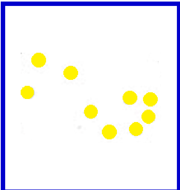
Escorpio
