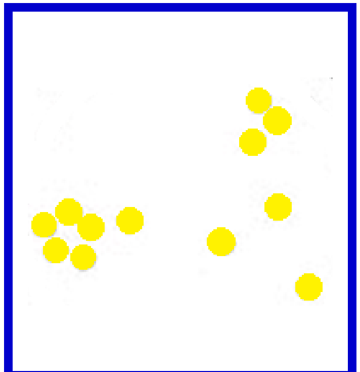
Piscis
