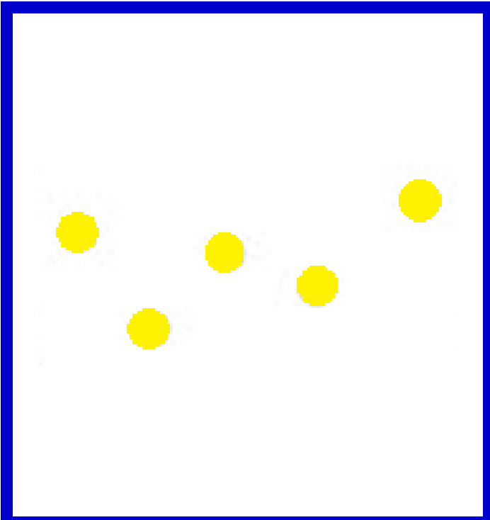
Casiopea
