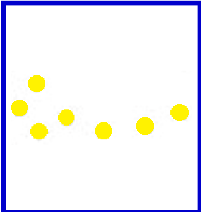
Osa Menor
