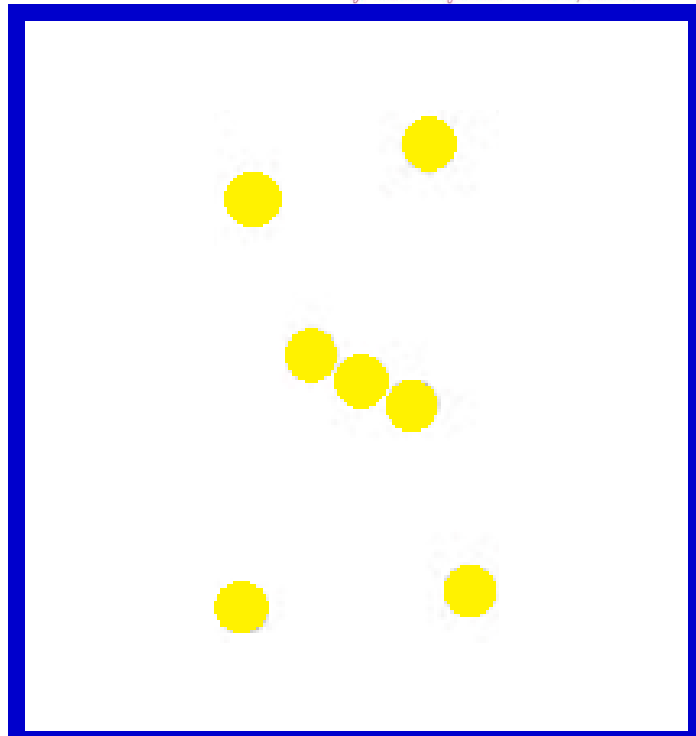
Orión
